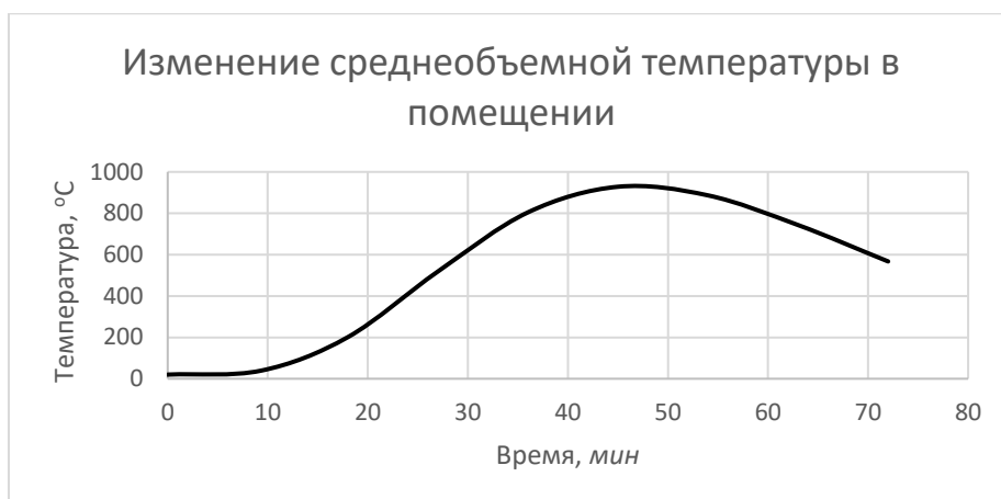
Рисунок 4.1 – Изменение среднеобъёмной температуры продуктов горения во времени
