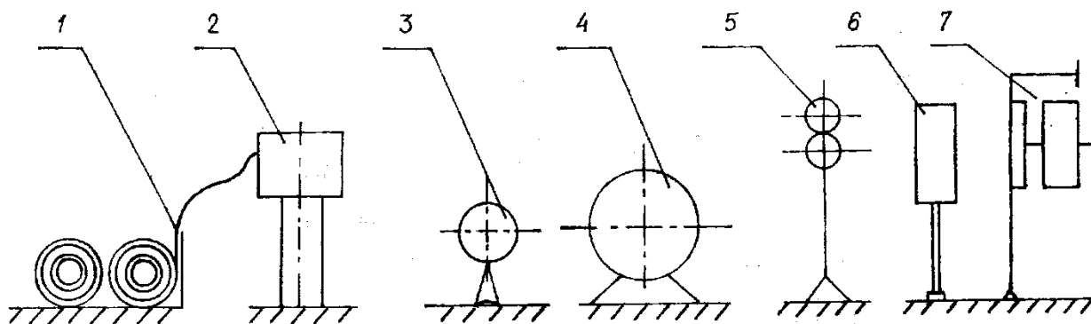
1 – ванна отмочки; 2 – рукавомоечная машина; 3 – накопительная катушка; 4 – агрегат для испытания, сушки и талькирования рукавов (АИСТ); 5 – приспособление для смотки рукавов; 6 – приспособление для ремонта рукавов; 7 – станок для навязки рукавов.
