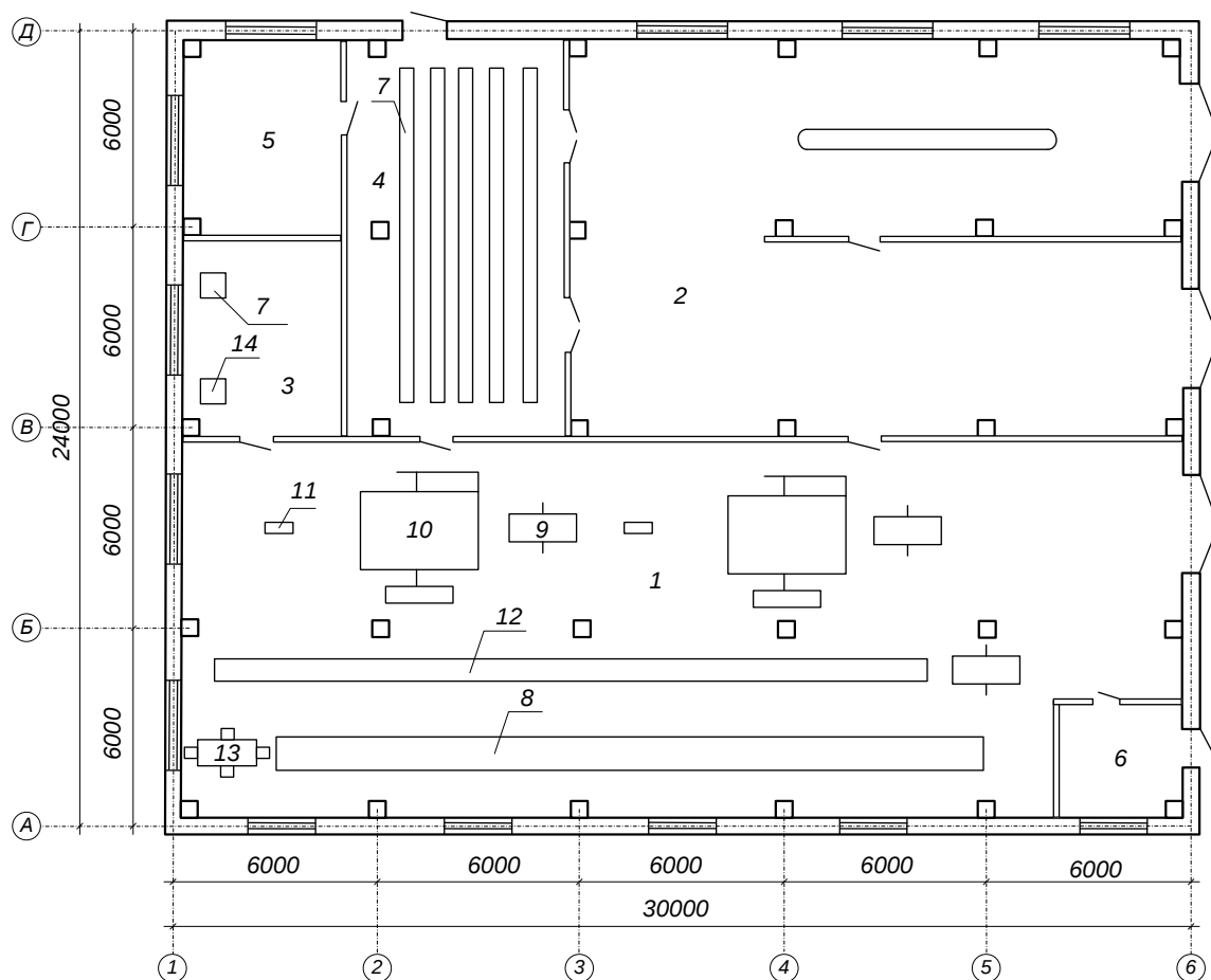
Примерная планировка централизованной рукавной базы
