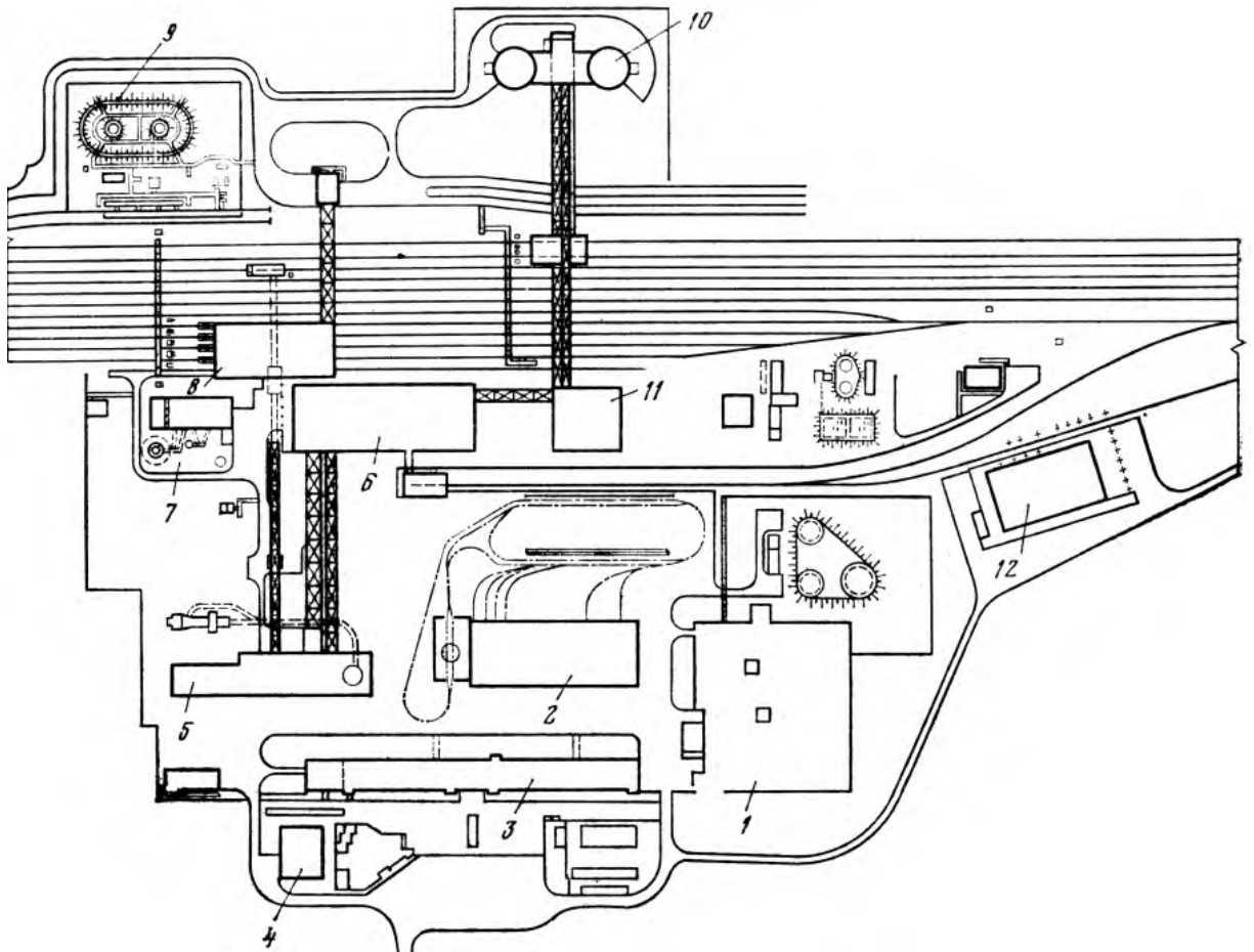
Рис. Генеральный план поверхности шахты:
