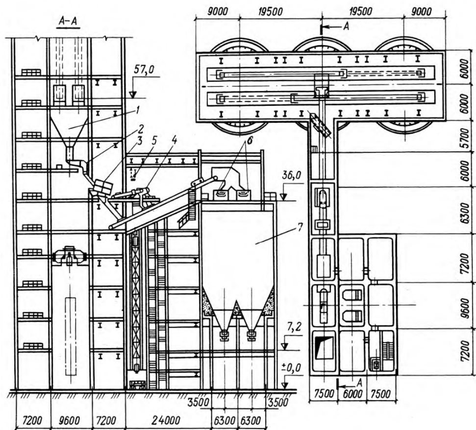
Рис. Блок технологического комплекса главного ствола:
