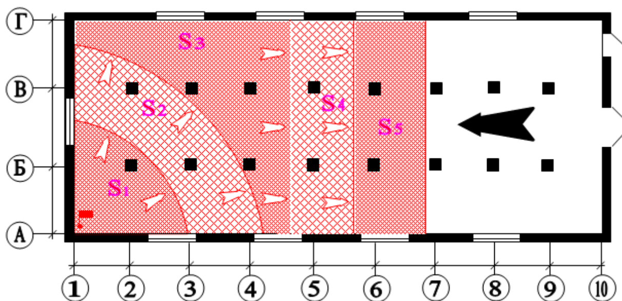
Рис. 2.4. План этажа с изображением обстановки возможного пожара на различные промежутки времени
