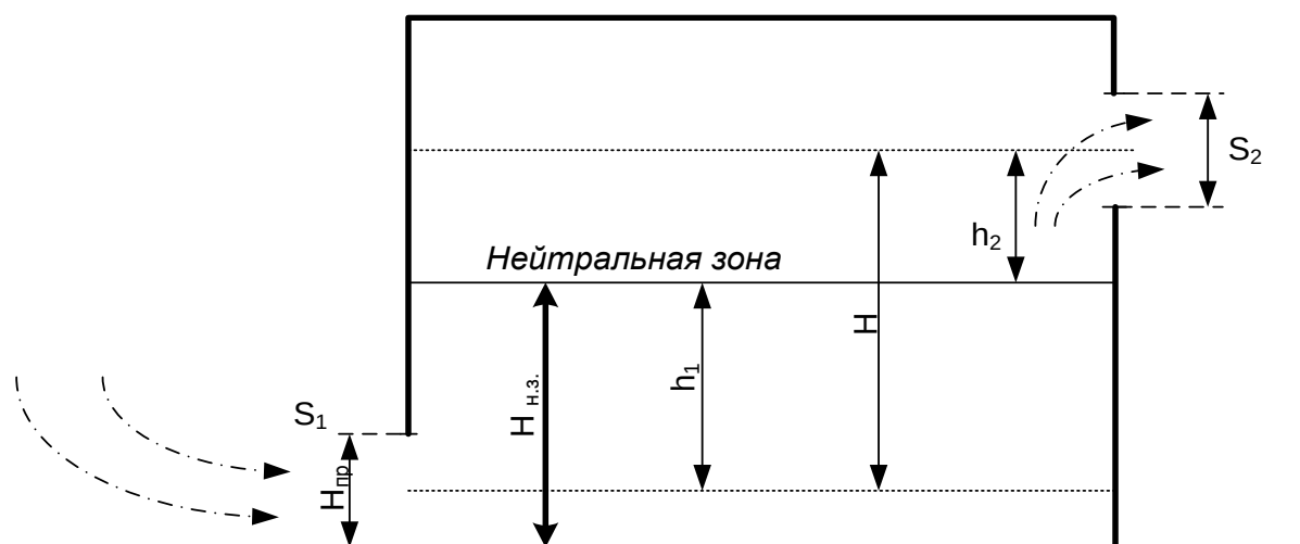
Рис. 2.1. Расположение нейтральной зоны при газообмене через проемы, расположенные на разной высоте
