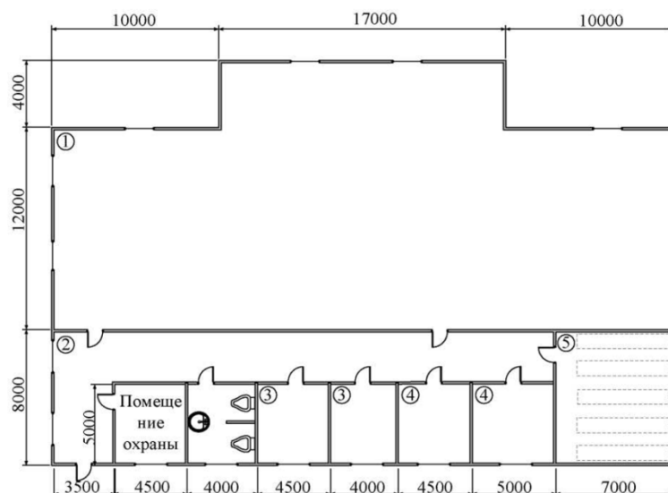
Объект №01- Одноэтажное здание швейной фабрики
